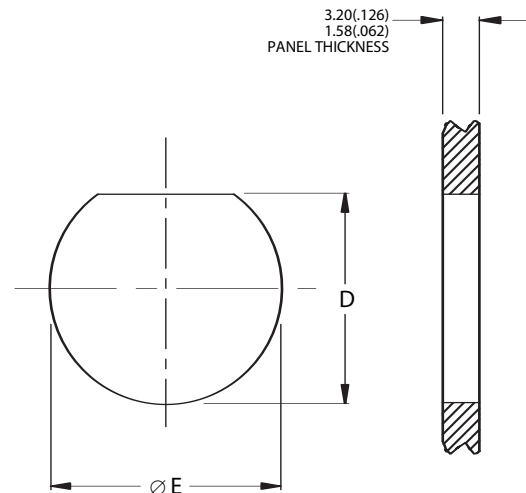
JAM NUT
